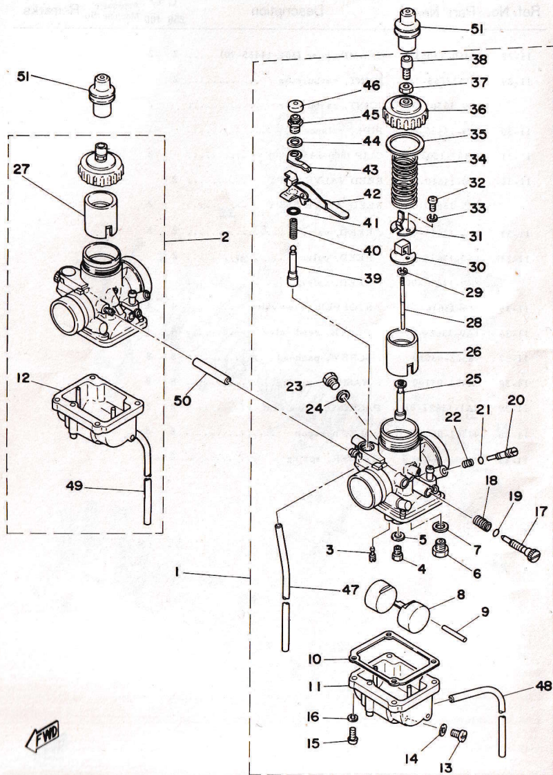
Fig. 12 CARBURETOR
