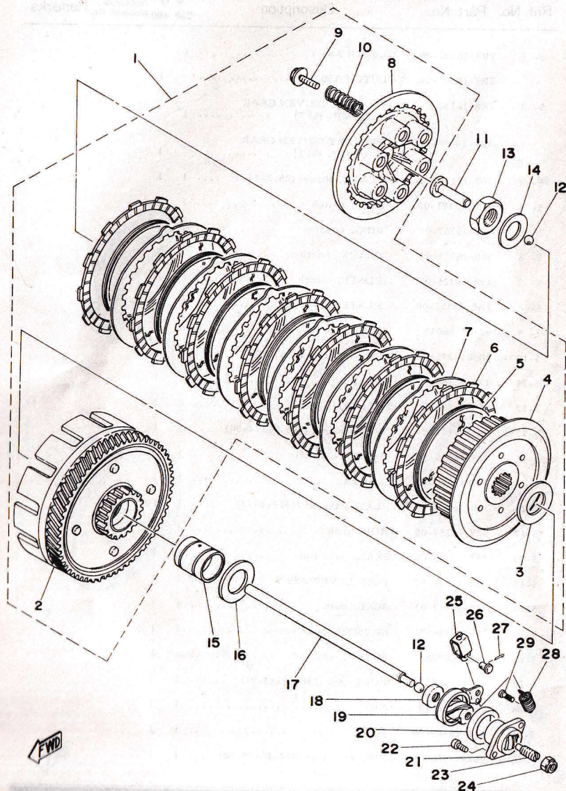
Fig. 5 CLUTCH
