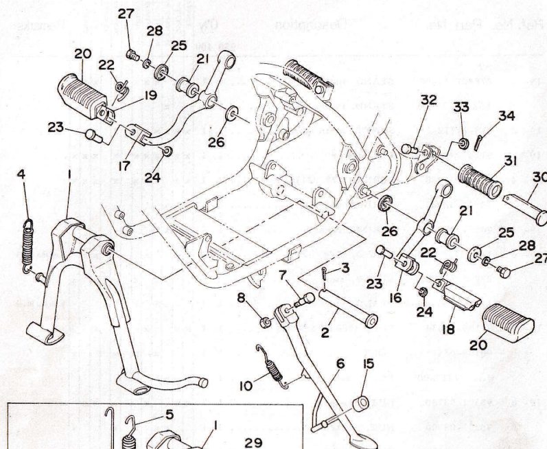
Fig. 19 STAND · FOOTREST
