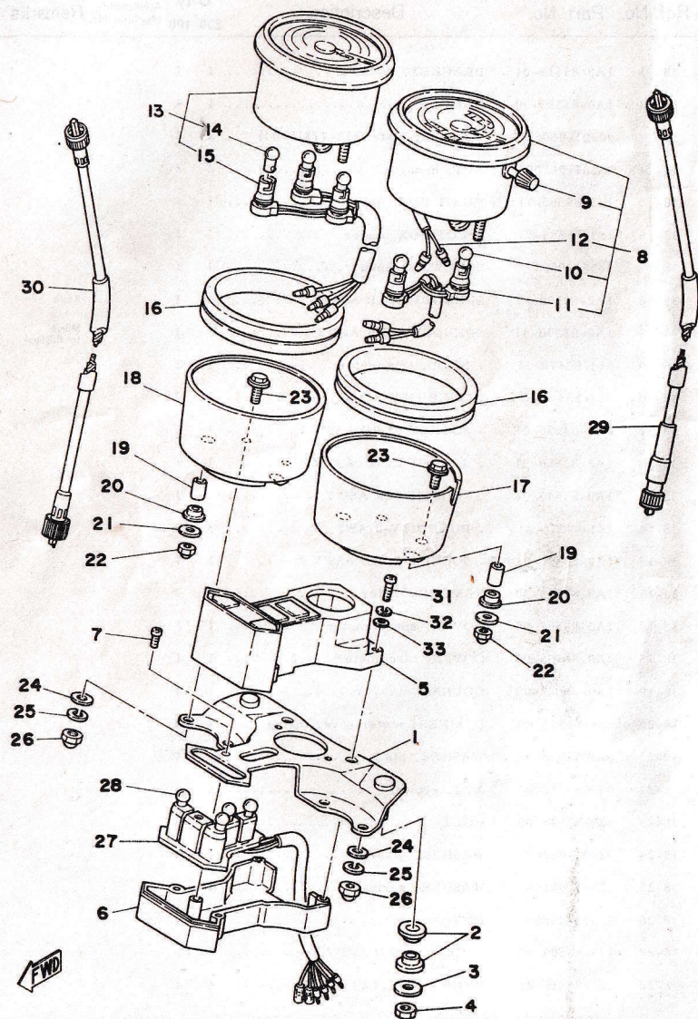
Fig. 38 SPEEDOMETER · TACHOMETER
