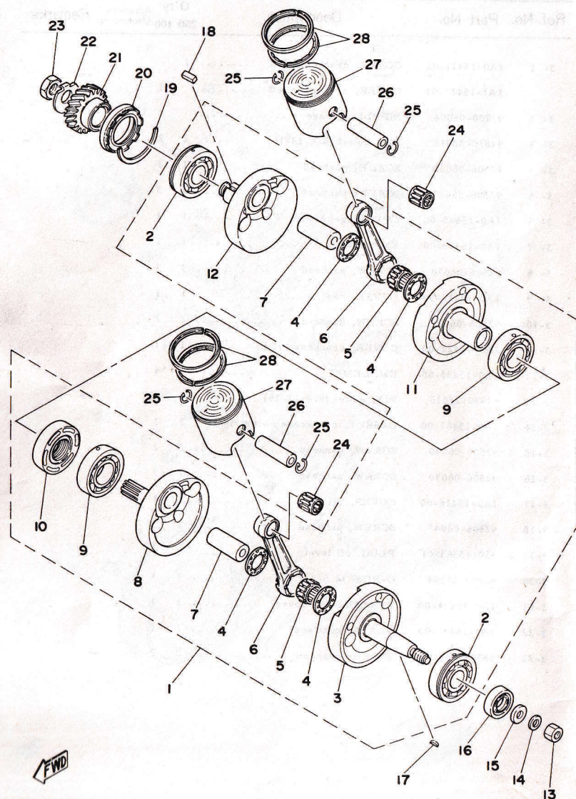
Fig. 4 CRANK · PISTON
