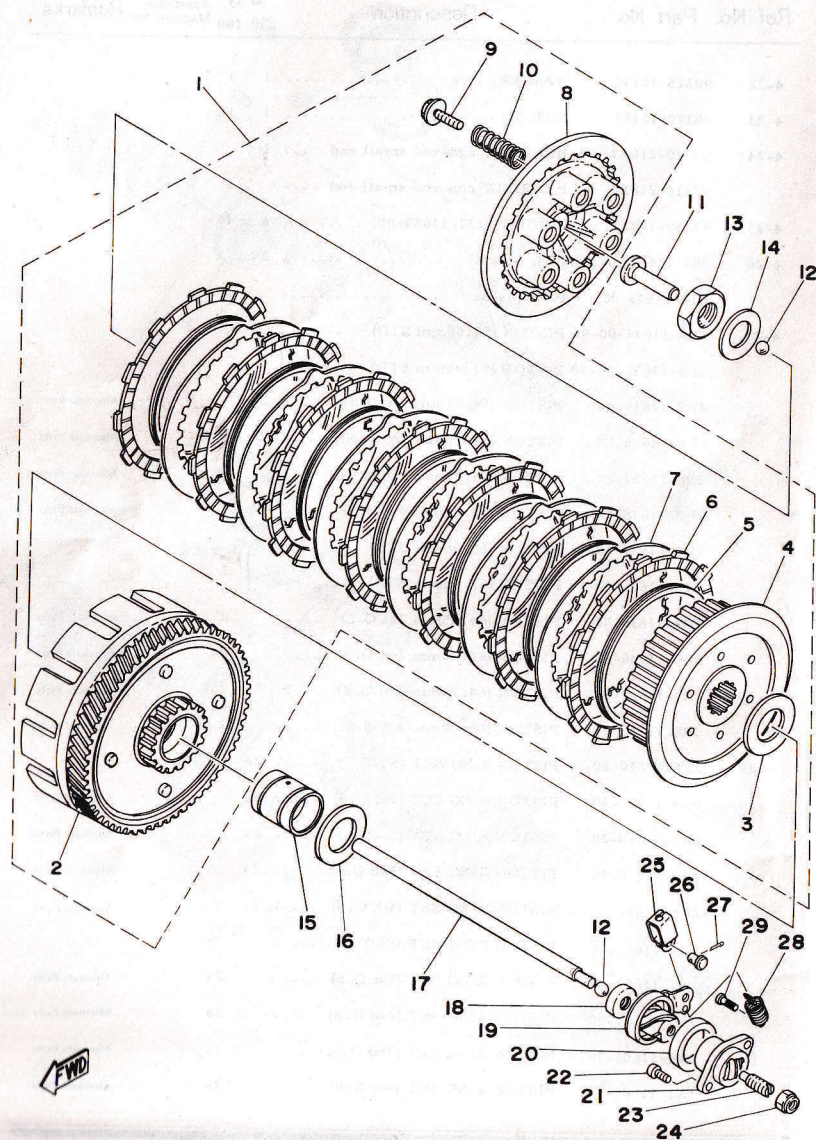
Fig. 5 CLUTCH
