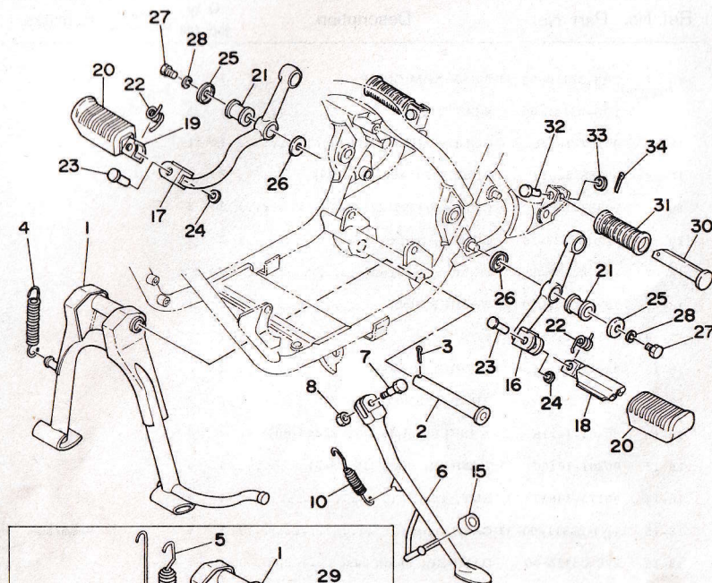
Fig. 19 STAND · FOOTREST
