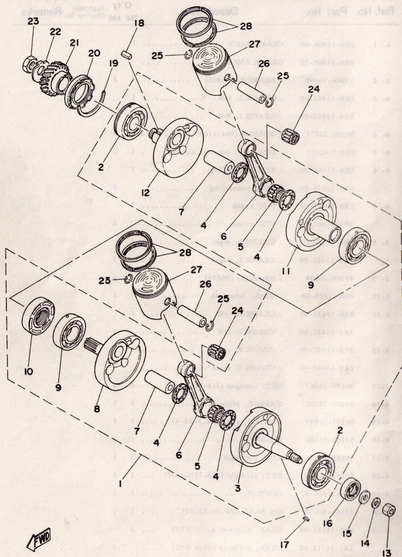
Fig. 4 CRANK · PISTON
