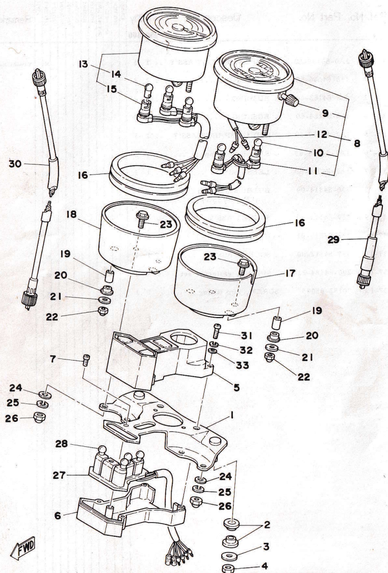
Fig. 38 SPEEDOMETER · TACHOMETER
