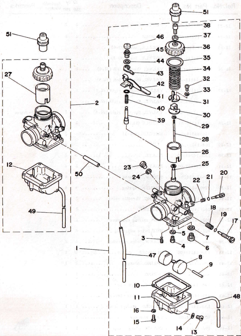
Fig. 12 CARBURETOR
