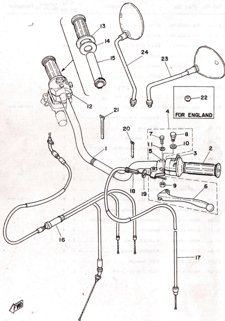
Fig. 24 HANDLE · WIRE
