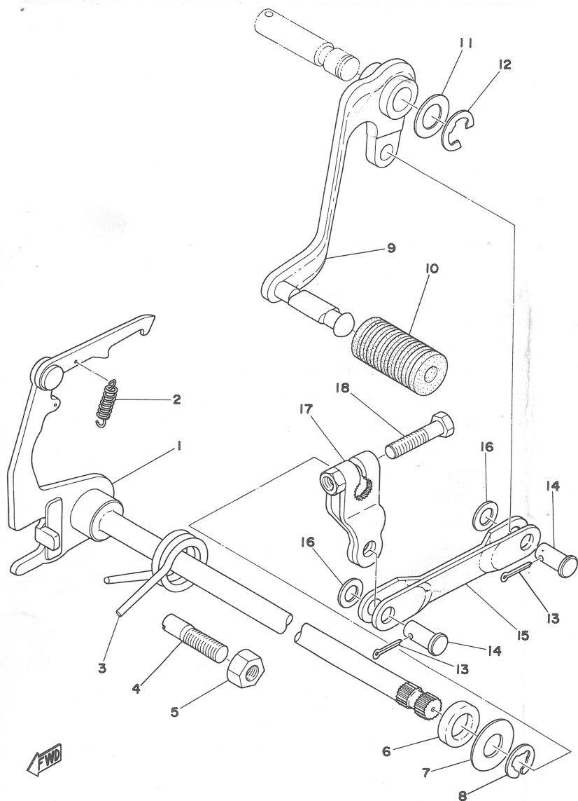
Fig. 7 SHIFTER 2
