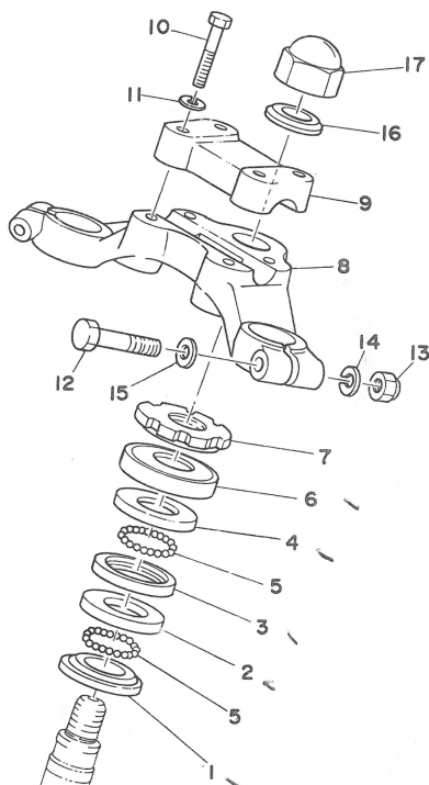
Fig. 22 STEERING
