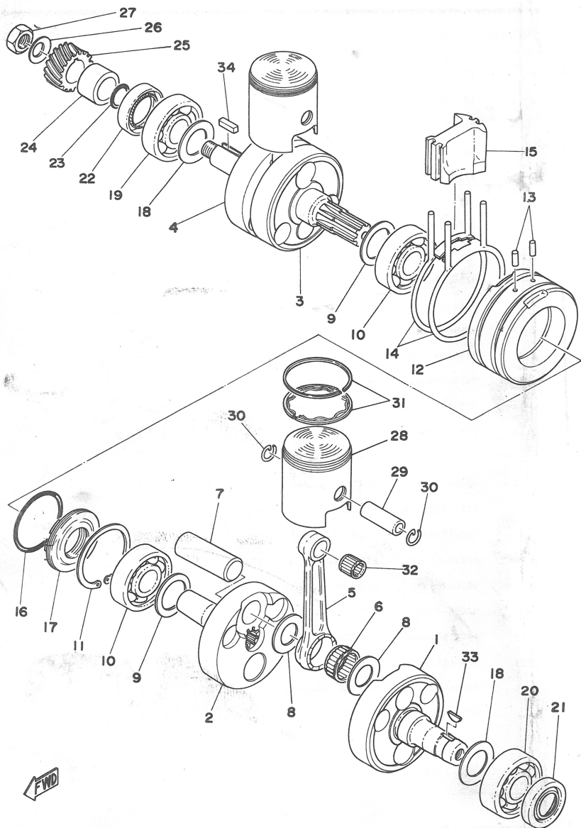
Fig. 3 CRANK · PISTON
