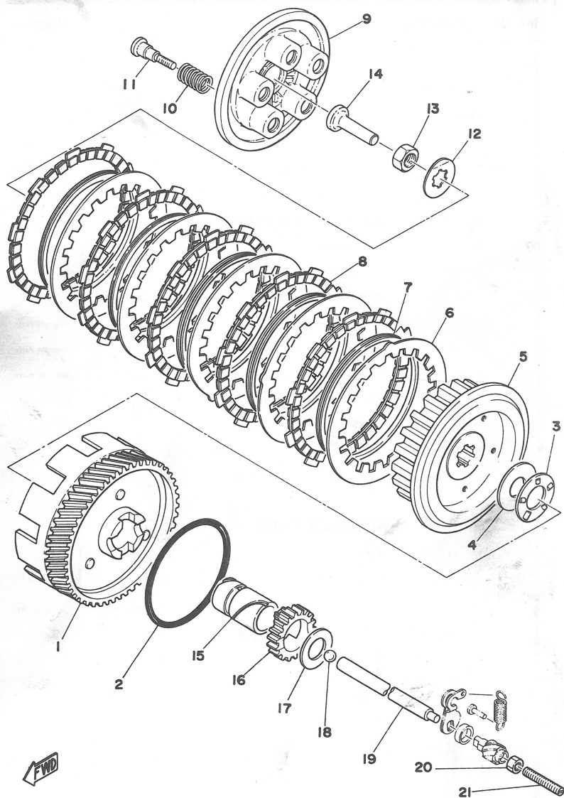
Fig. 4 CLUTCH
