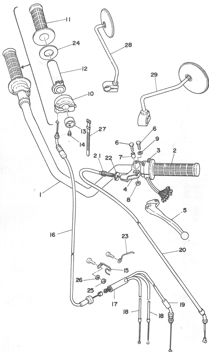
Fig. 24 HANDLE · WIRE
