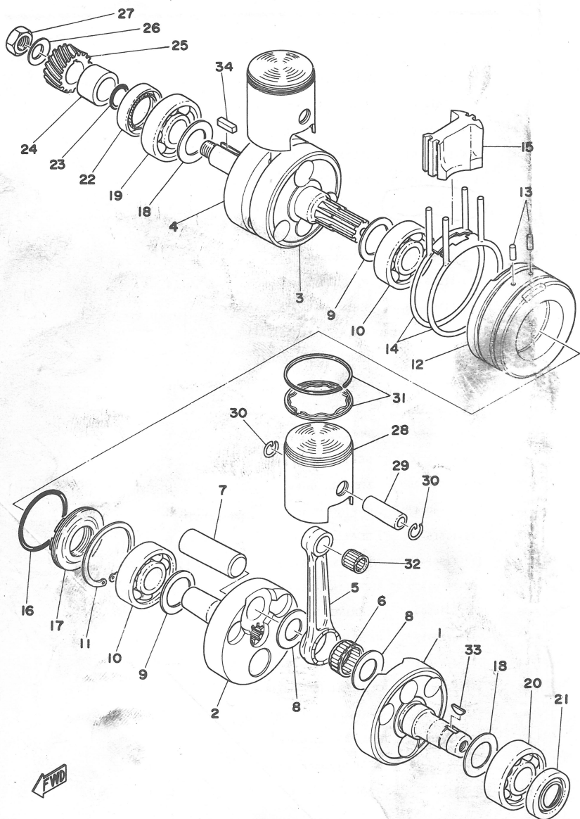
Fig. 3 CRANK · PISTON
