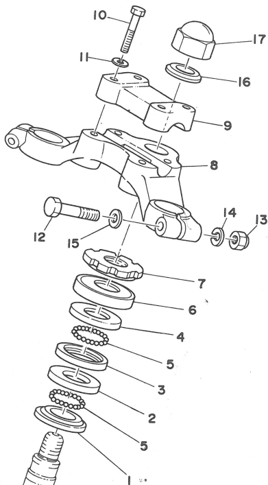
Fig. 22 STEERING
