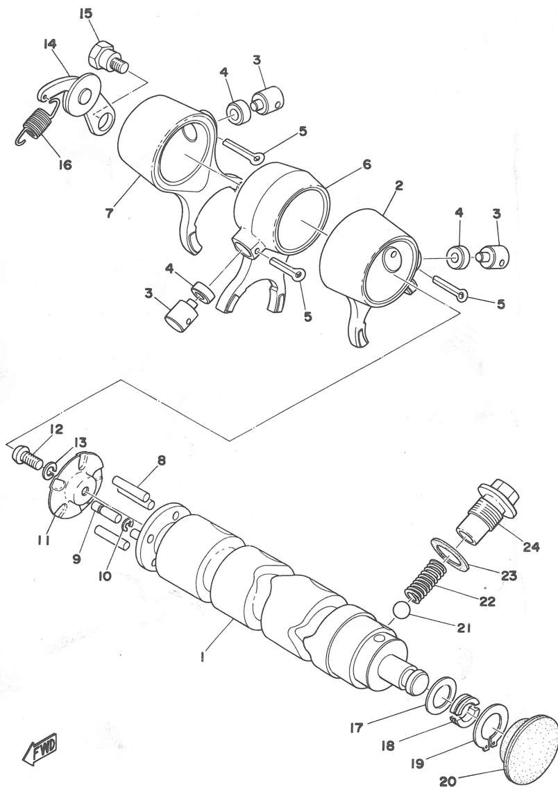
Fig. 6 SHIFTER 1
